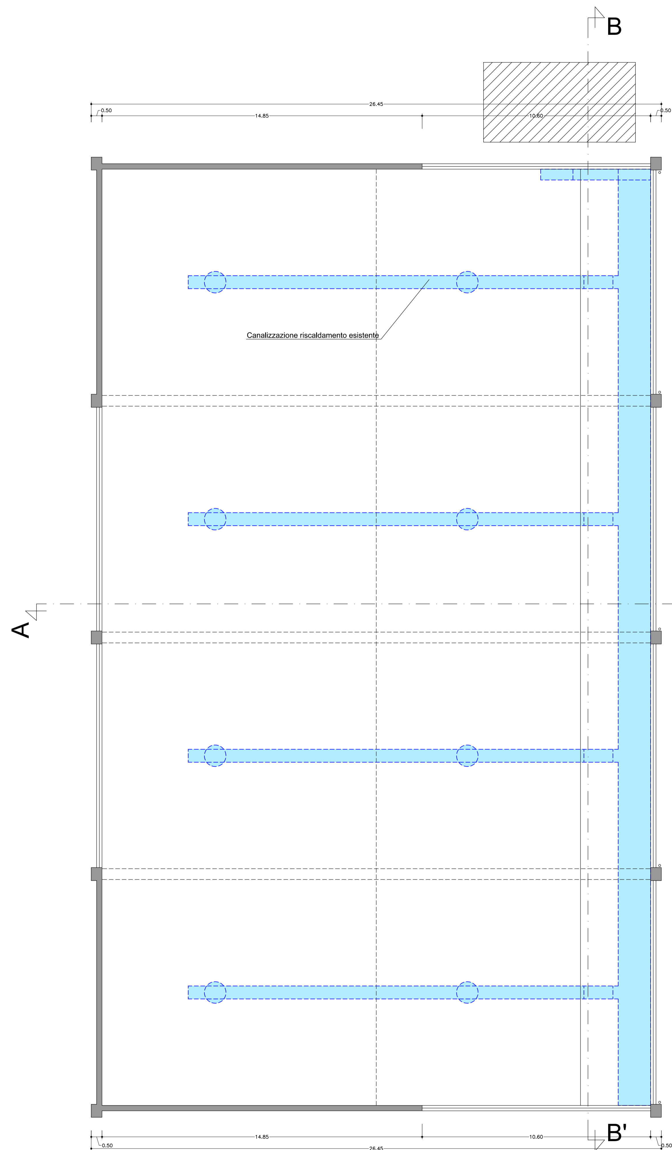
PIANTA - Livello finestratura palestra -
